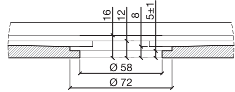
DETTAGLIO BUCO SIFONE - V
